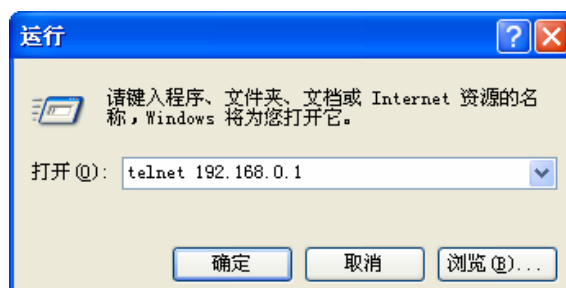
图 1-9 运行窗口
