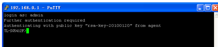
图 1-24 登录交换机
