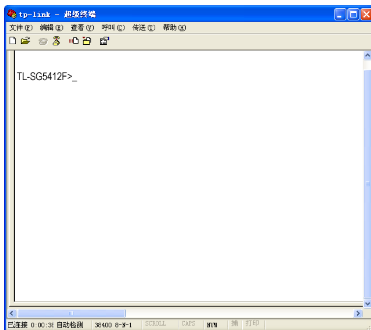
图 1-5 登录交换机
