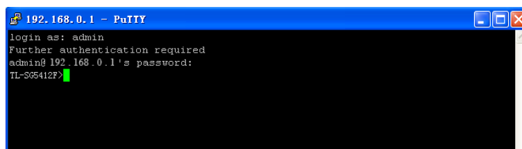
图 1-18 登录交换机
